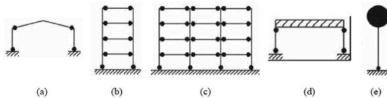
Figura C7.5.1 - Configurazioni dissipative di strutture intelaiate: disposizione delle cerniere plastiche, secondo le tipologie esposte nella Tabella 7.3.11 del § 7.3.1 delle NTC
