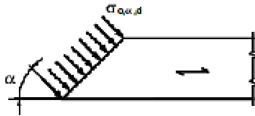
Figura 6-2 –Tensioni inclinate rispetto alla fibratura
